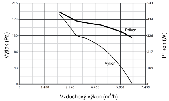
A-E 506 M
