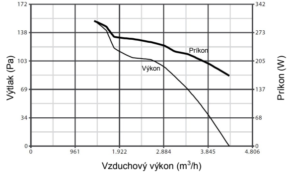
A-E 454 M
