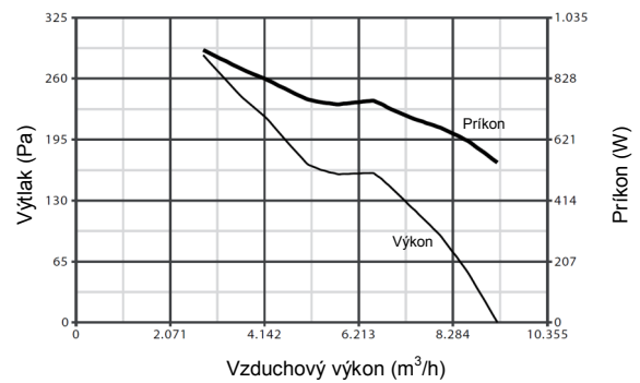
A-E 564 T
