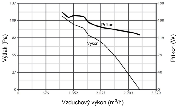
A-E 404 T
