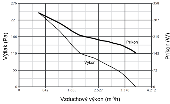
A-E 454 T
