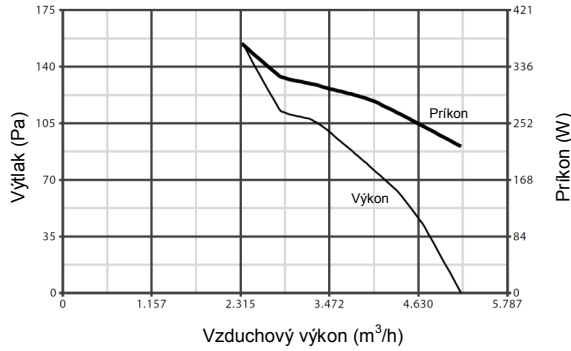
A-E 504 T
